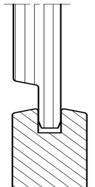
38 mm deur strak bossingspaneel
