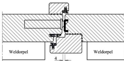
T54-3 Houten slaglatten 54 mm binnendraaiend
