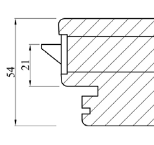
Aanslag dagschoot 54 mm detail D/E
