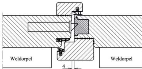
T54-2 Houten slaglatten bij Buva Ergo-Duo 54 mm binnendraaiend
