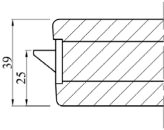
Aanslag dagschoot stomp 38/40 mm
