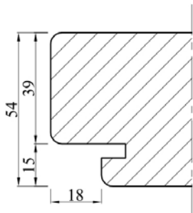
54 mm kaderdetail A
