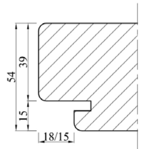
54 mm kader AR (3-zijdig 18x15A en onder 15x15R)
