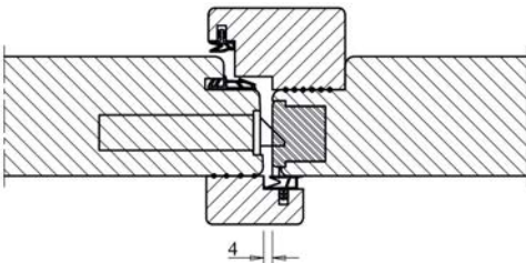
T54-5 Houten slaglatten bij Buva Ergo-Duo 54 mm buitendraaiend
