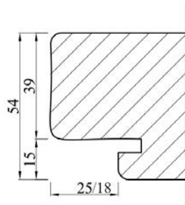
54 mm kaderdetail F (3-zijdig 25x15 en onder 18x15)
