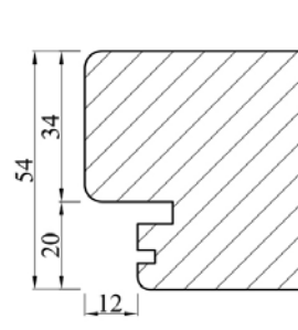
54 mm kaderdetail D
