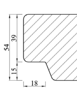
54 mm verjonging detail B buiten
