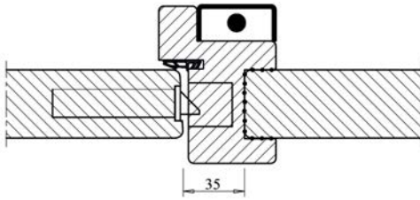
T40-4 Houten tongstijl met Buva 8034 38/40 mm buitendraaiend
