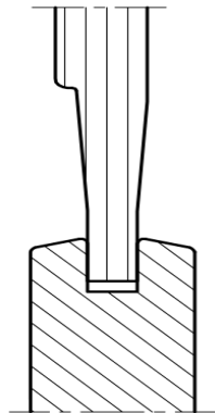
38 mm deur traditioneel bossingspaneel
