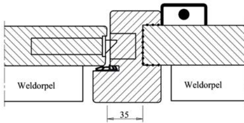
T40-1 Houten tongstijl met Buva 8012 38/40 mm binnendraaiend
