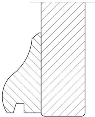
Weldorpel
