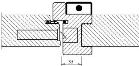
T54-4 Houten tongstijl met Buva 8034 54 mm buitendraaiend met kaderdetail A
