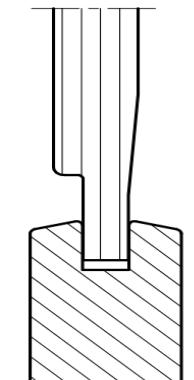
38 mm deur gegroefd paneel
