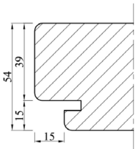
54 mm kaderdetail R
