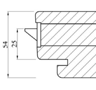
Aanslag dagschoot 54 mm detail A
