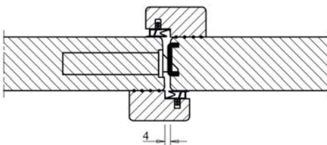
T40-6 Houten slaglatten 38/40 mm buitendraaiend
