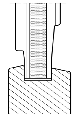
54 mm deur gegroefd paneel
