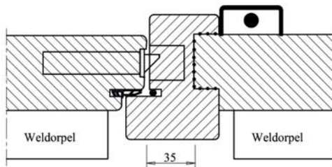
T54-1 Houten tongstijl met Buva 8012 54 mm binnendraaiend met kaderdetail A
