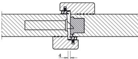
T40-5 Houten slaglatten bij Buva Ergo-Duo 38/40 mm buitendraaiend
