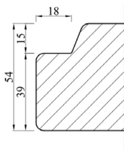
54 mm verjonging detail C binnen
