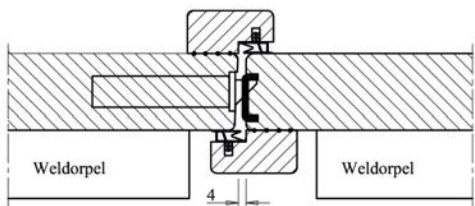
T40-3 Houten slaglatten 38/40 mm binnendraaiend
