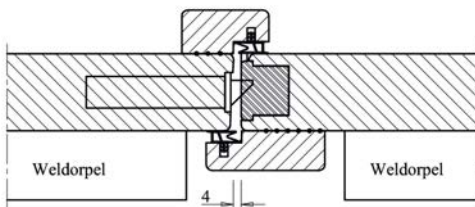
T40-2 Houten slaglatten bij Buva Ergo-Duo 38/40 mm binnendraaiend
