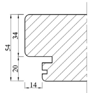
54 mm kaderdetail E
